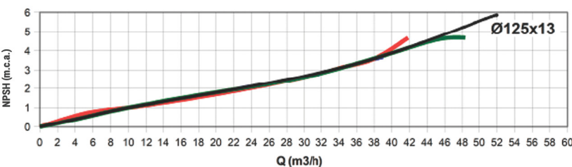
ALTURA MANOMETRICA (m.c.a.)
